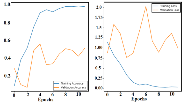
ResNetRS101
