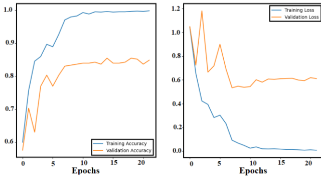
EfficientNetV2B0
