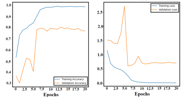
RegNetY032
