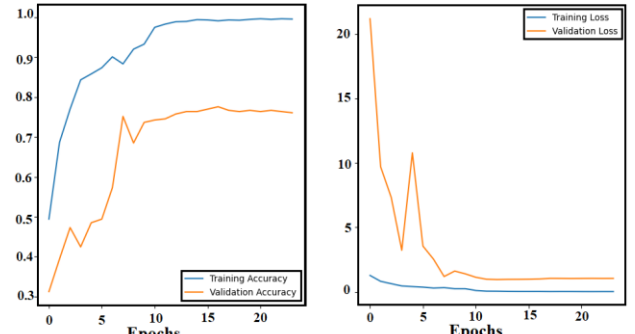
XceptionNet
